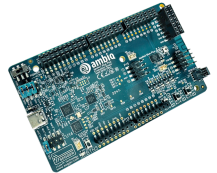
Apollo3 Blue Plus AMA3B2EVB (EVB)
